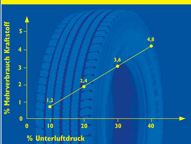
Einfluss des Luftdrucks auf den Kraftstoffverbrauch
