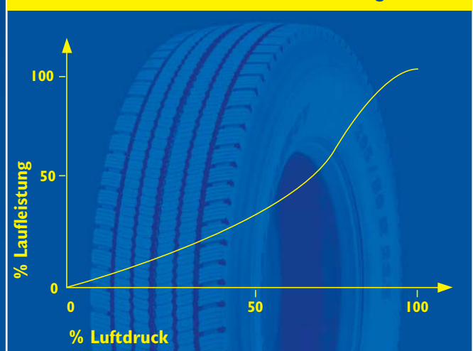
Einfluss des Luftdrucks auf die Laufleistung
